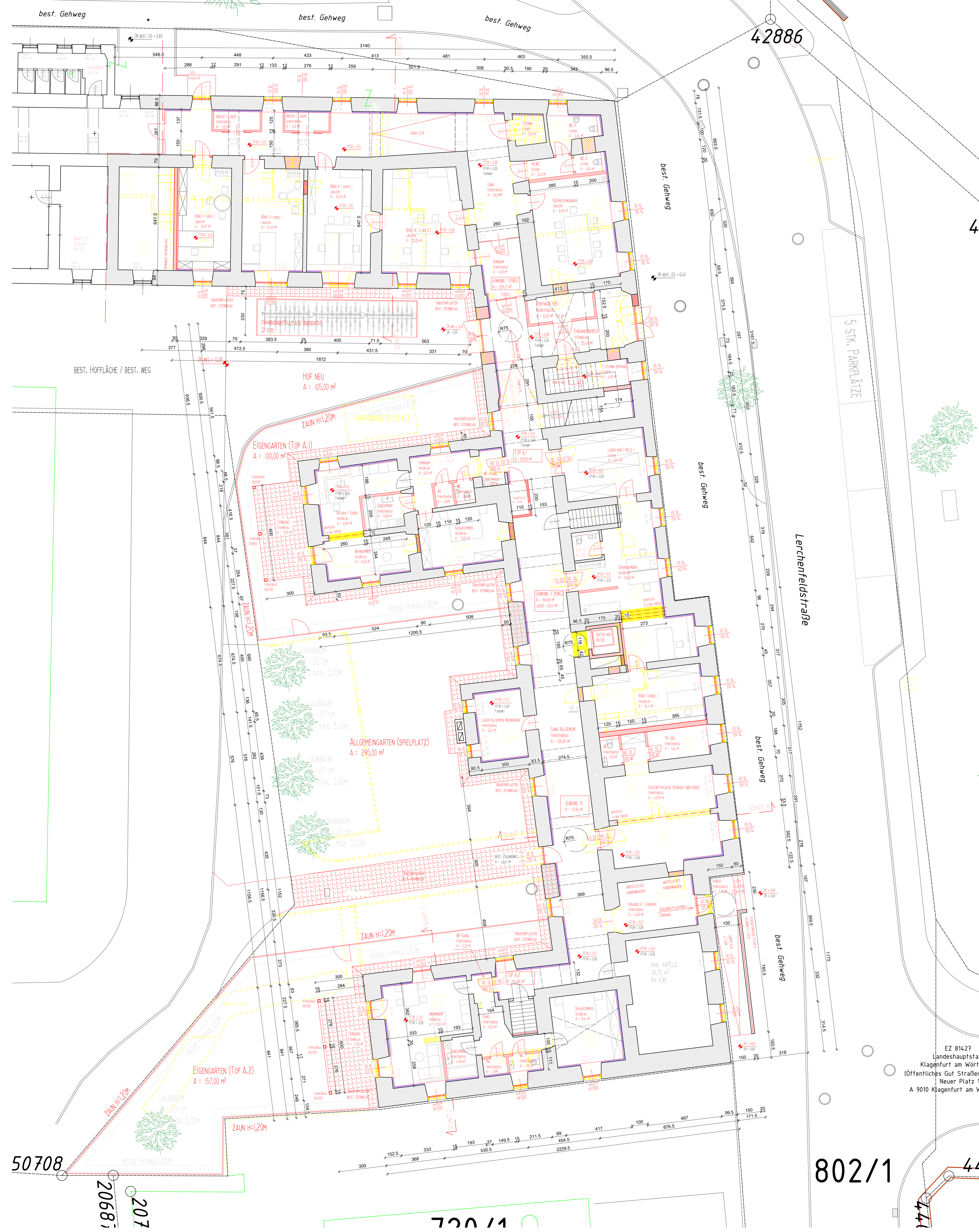
Grundriss Erdgeschoss M 1/100
