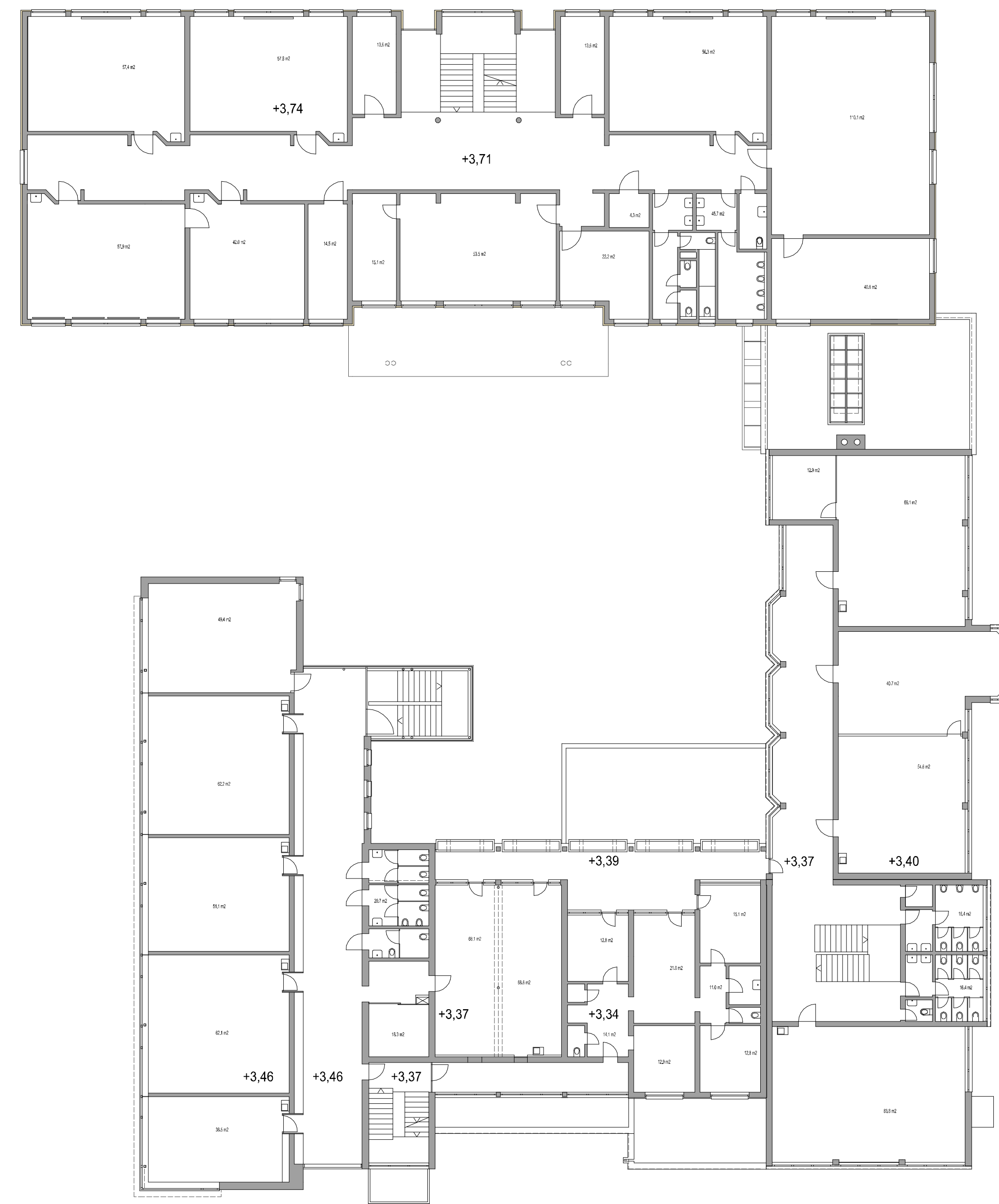
Obergeschoß 597 + 759 m2
