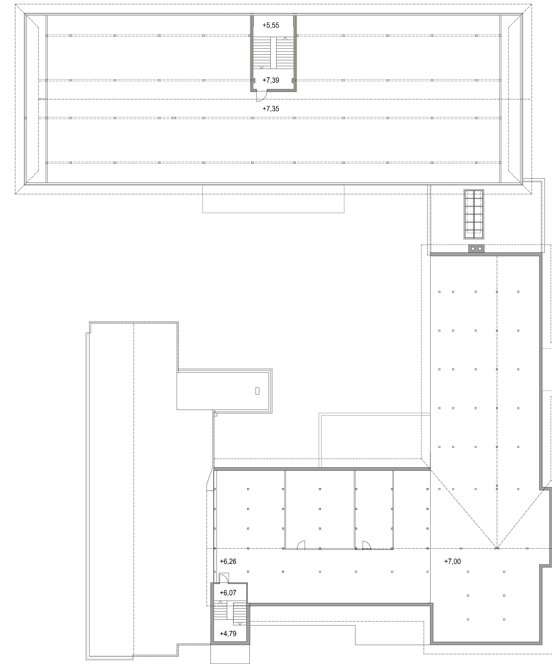
Dachgeschoß
