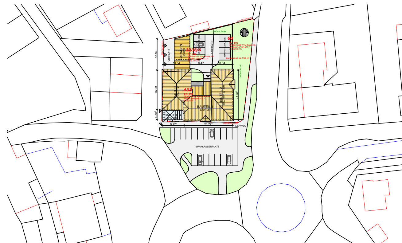
Grundriss Außenanlagen
