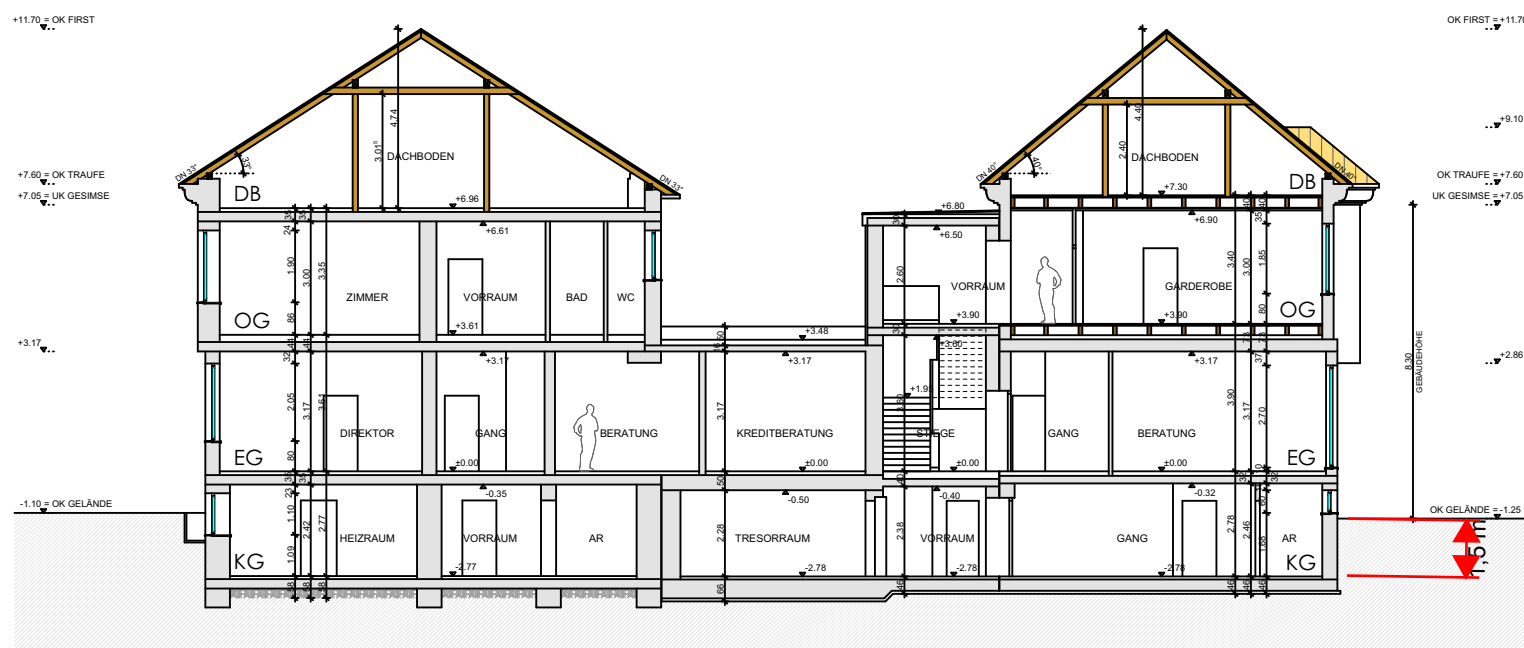
Schnittdarstellung
