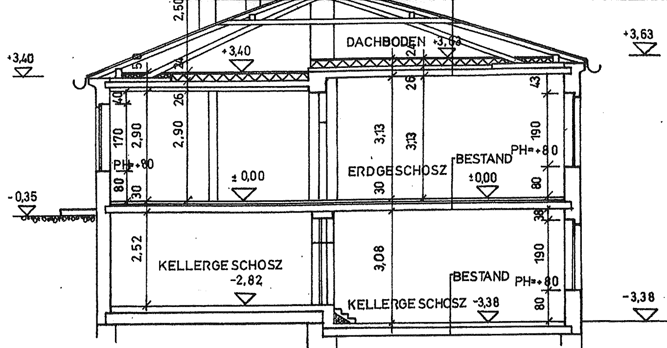
SCHNITT A-B 1:100
